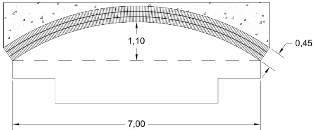
secció S1 (T5)
